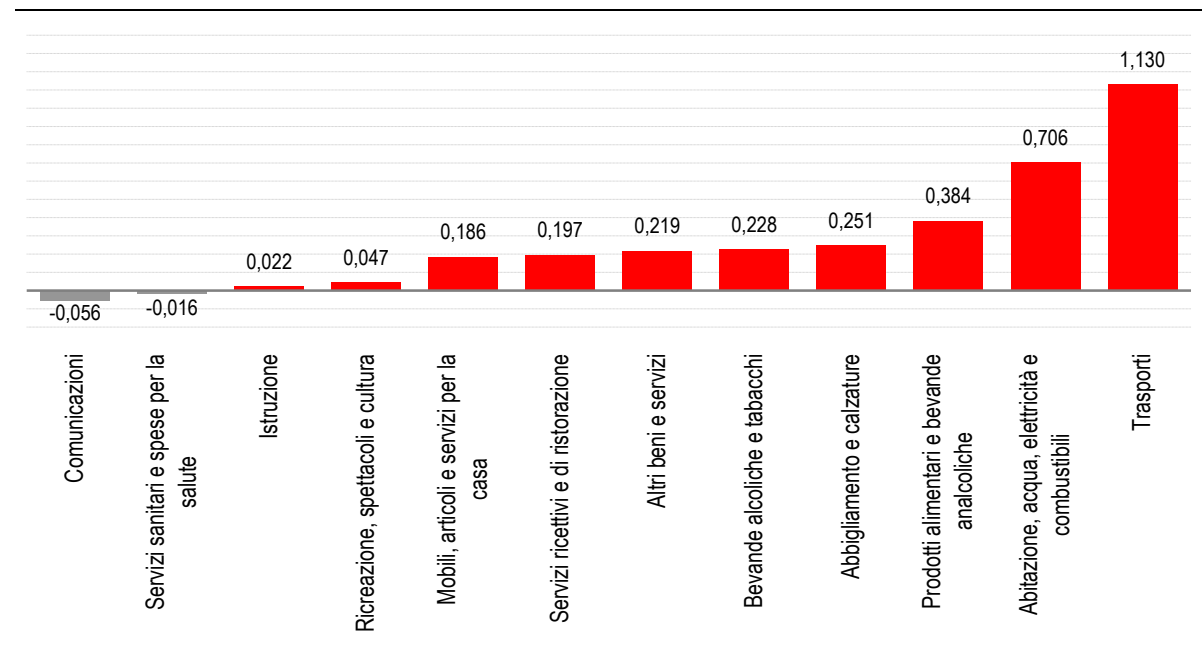
FIGURA 3. INDICI DEI PREZZI AL CONSUMO NIC, PER DIVISIONE DI SPESA Aprile 2012, contributo alla variazione tendenziale dell'indice generale
